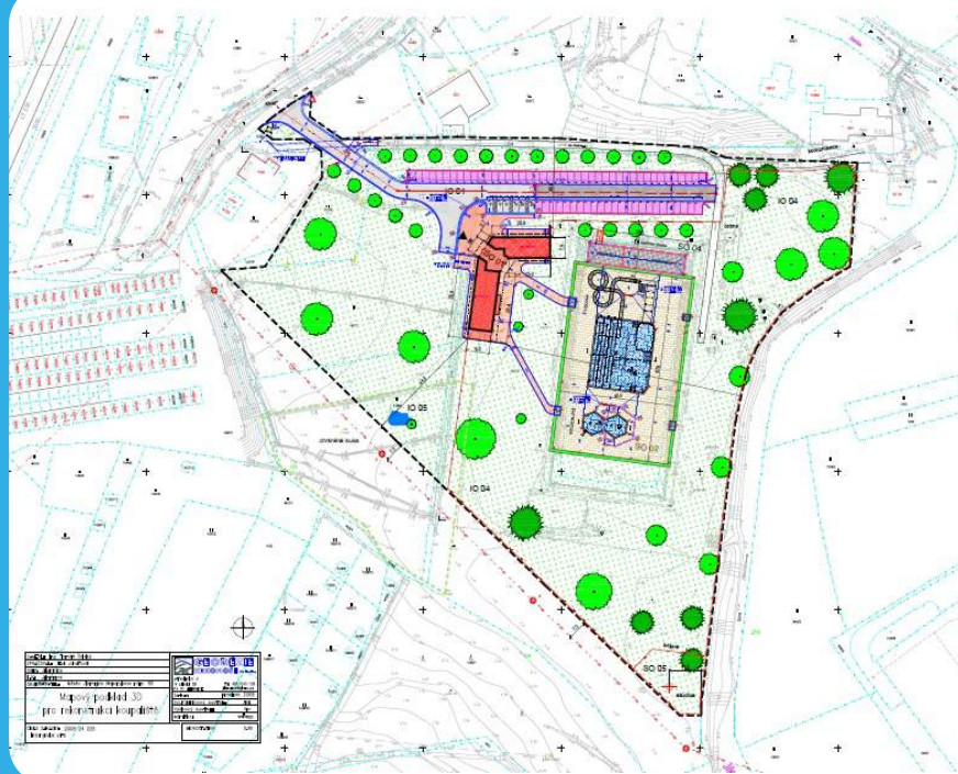
situace koupaliště, zpracoval ing. Milan Šmíd
