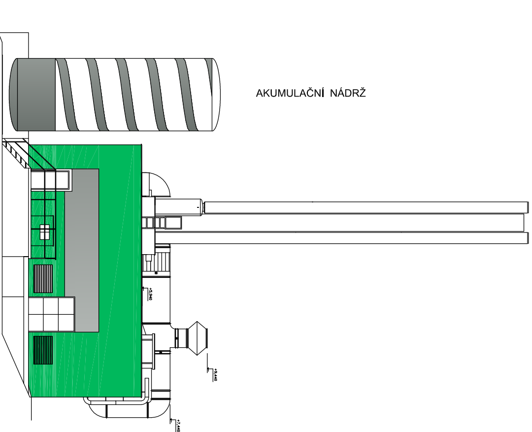
POHLED VÝCHODNÍ 1:200
