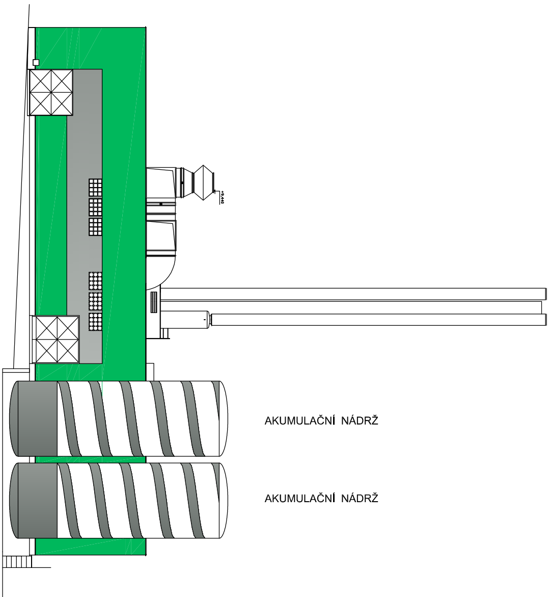
POHLED JIŽNÍ 1:200
